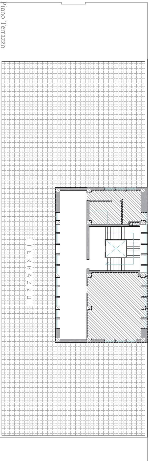
Pianta Piano Rialzato
